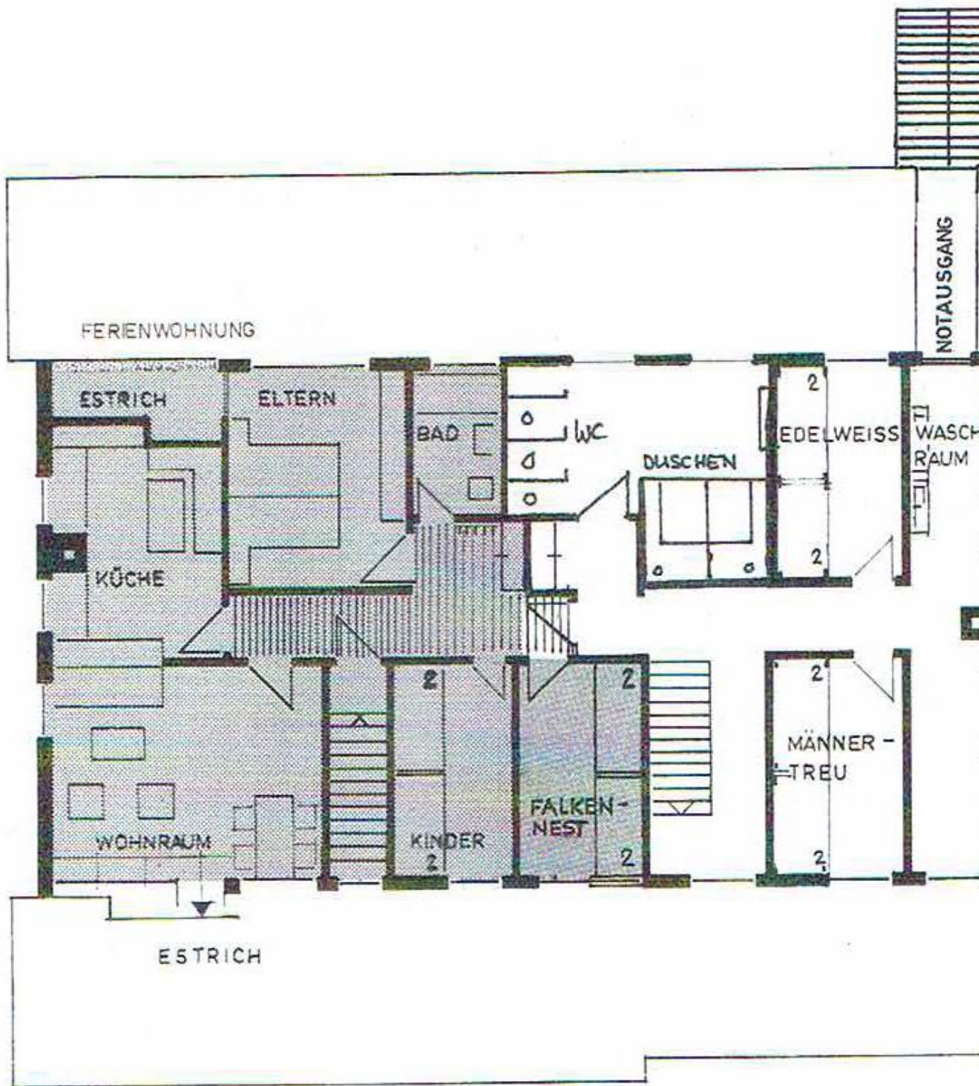
Grundriss Dachgeschoss
